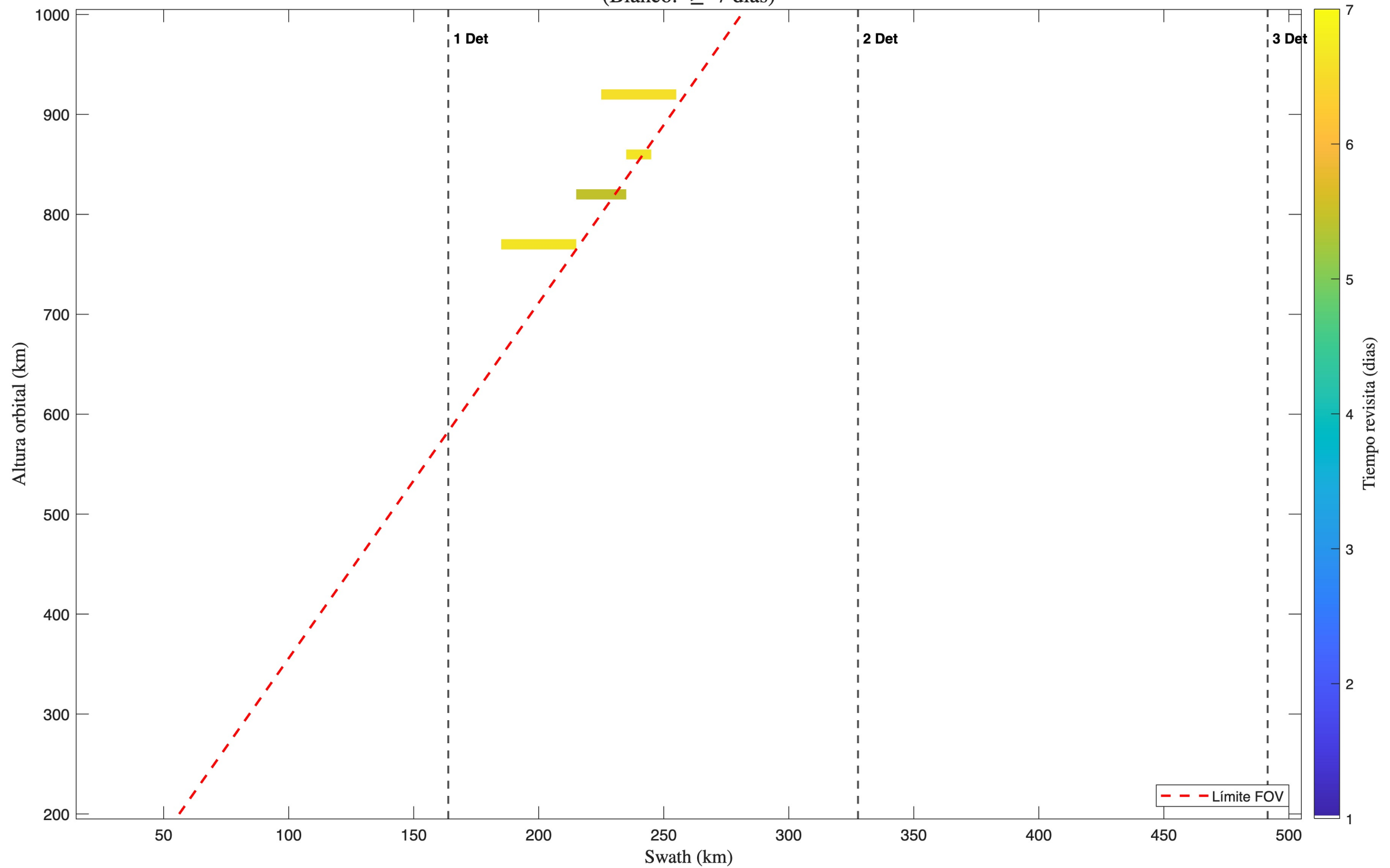
Tiempo Revisita - 2 Satelite(s); 2 Telescopio(s): TMA; Detector 2 (Blanco: \geq 7 dias)
